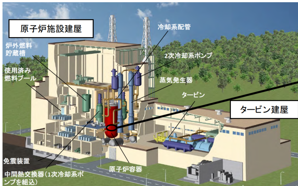
高速炉システムの鳥瞰図例
