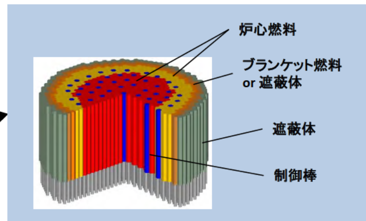
炉心(原子炉容器の中にある)
